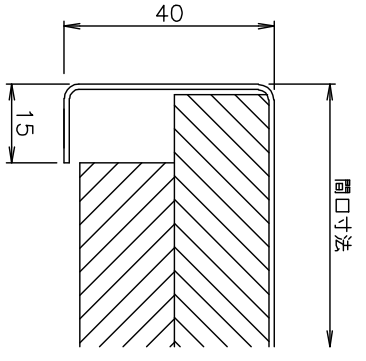
面端コ曲げ断面
