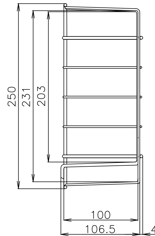
断面B-B
