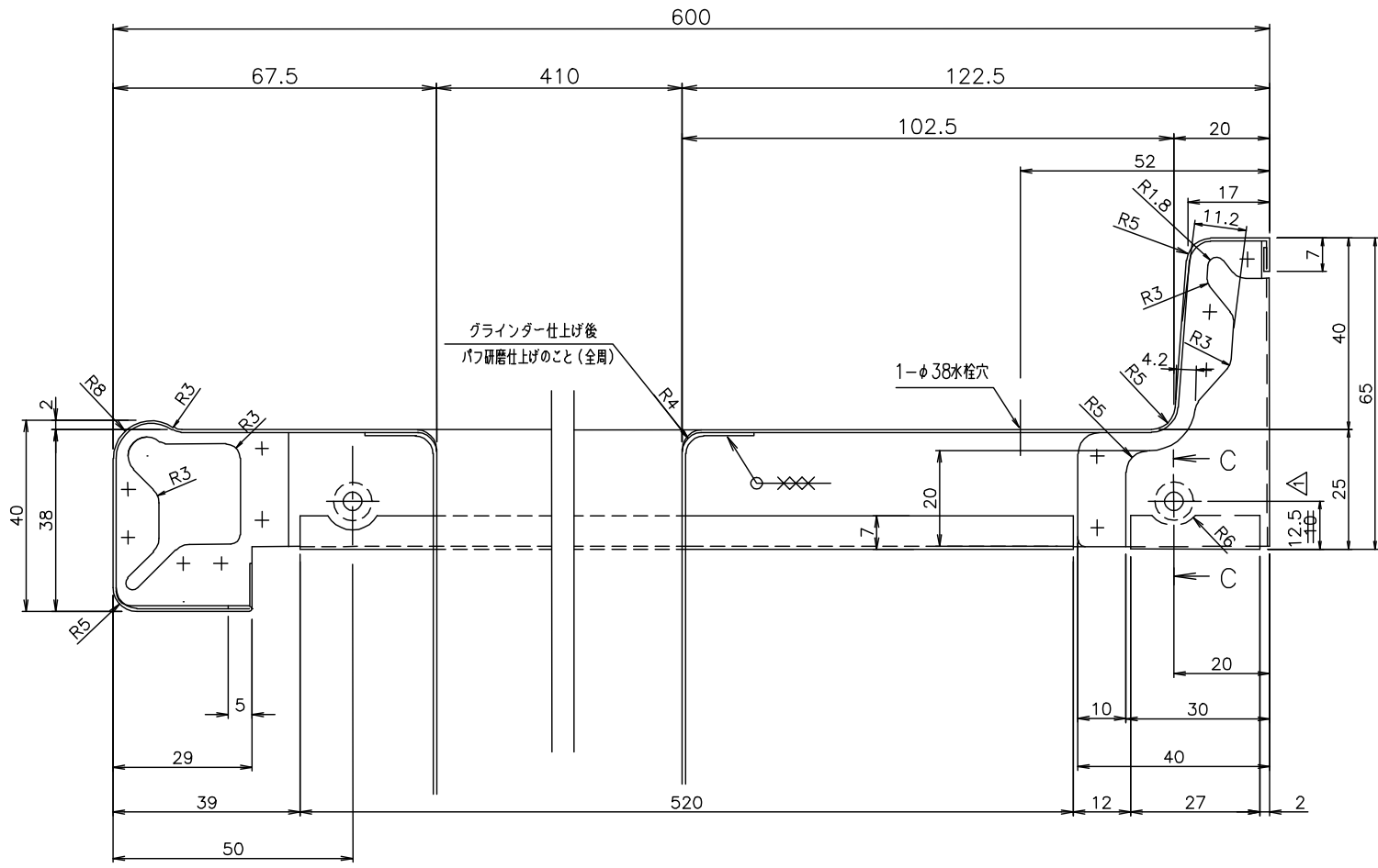
A-A断面図(1/1)
