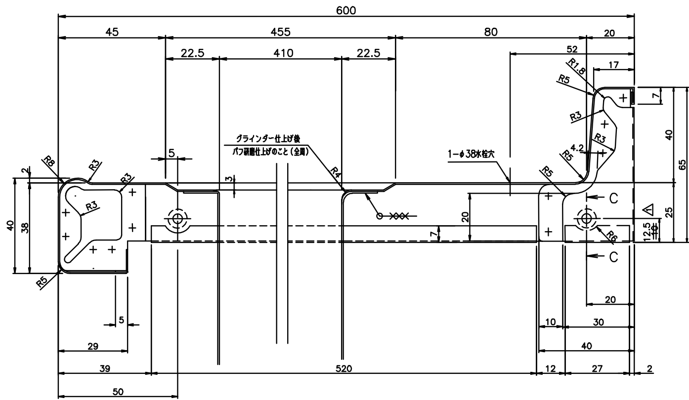
A-A断面図(1/1)
