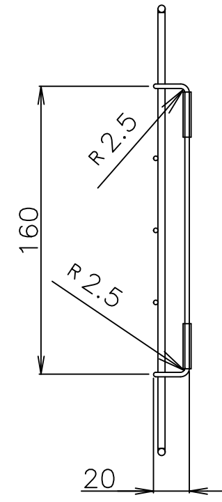
断面 A-A
