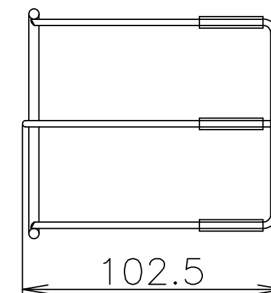
断面A-A
